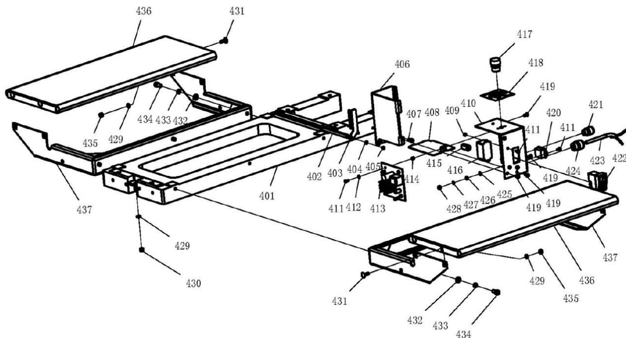
Чертеж № 4 Расширители рабочего стола
