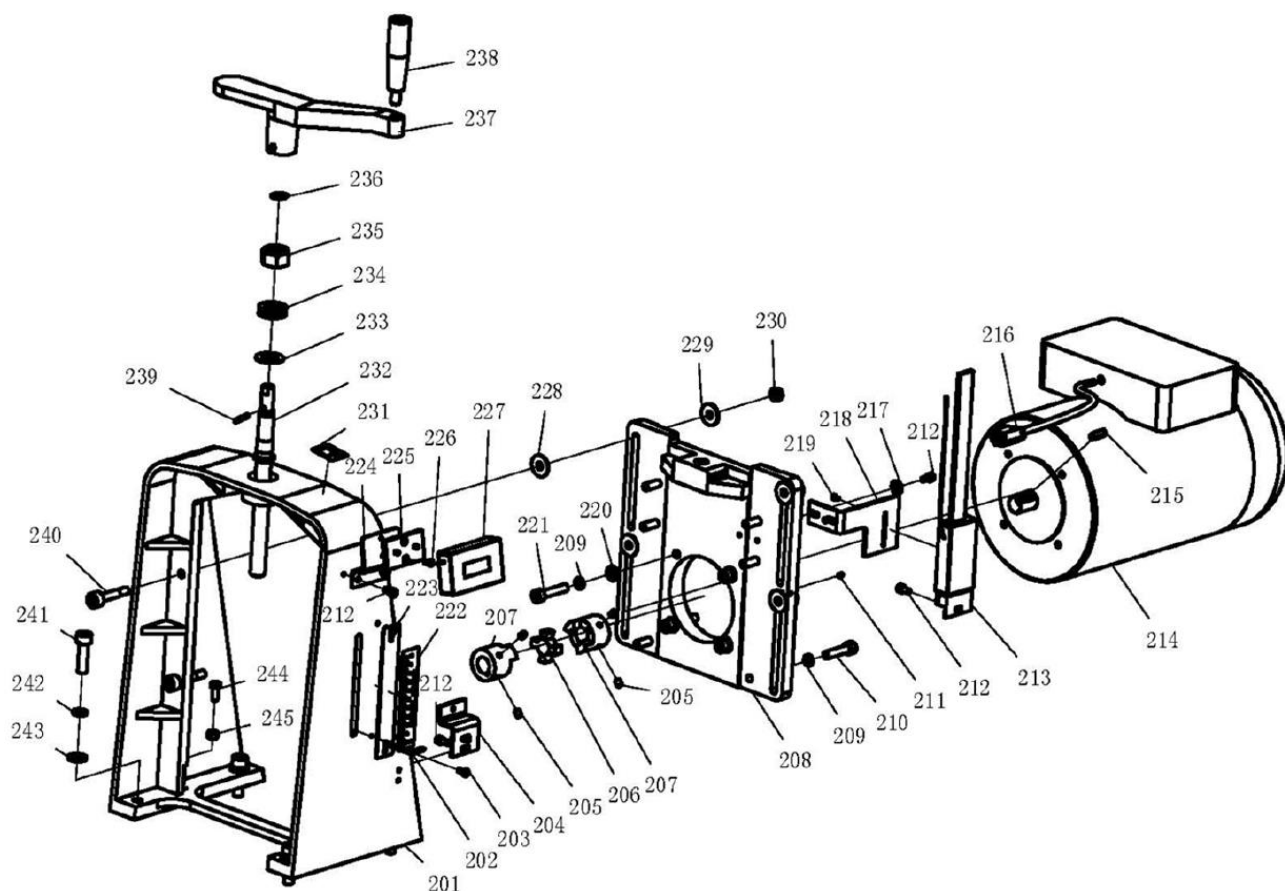
Чертеж №2 Корпус крепления шлифовального барабана
