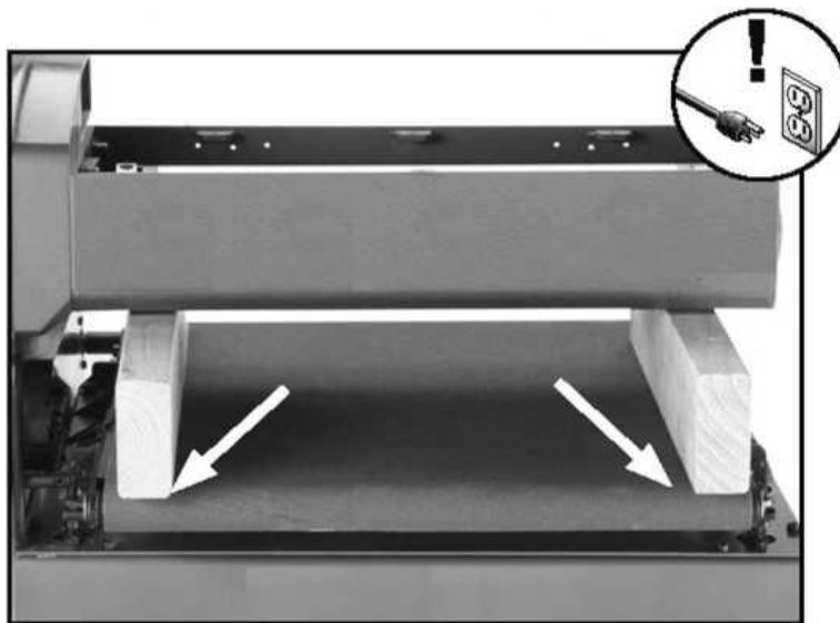
Рисунок 46. Пример калибровочных блоков (брусочей), размещенных под барабаном.
