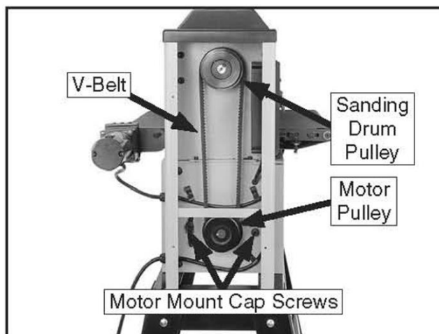
Рисунок 38 Система ременной передачи
